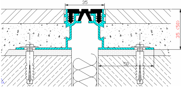
DL 1A 35*35 DL 1A 35*50
