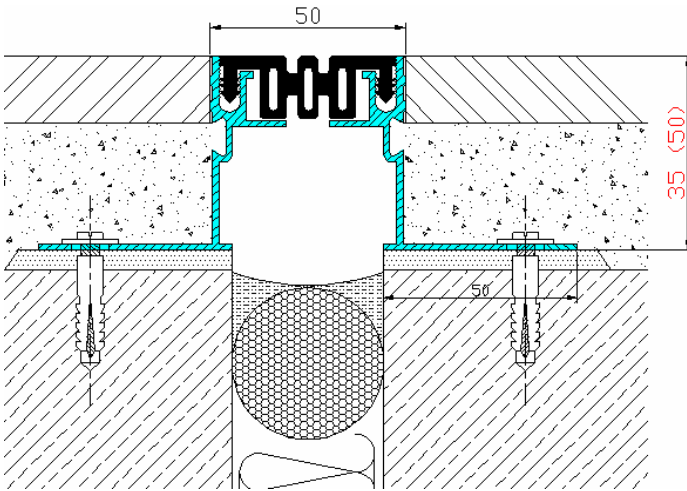
DL 1A 50*35 DL 1A 50*50
